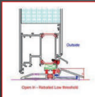
DOOR CROSS SECTION
